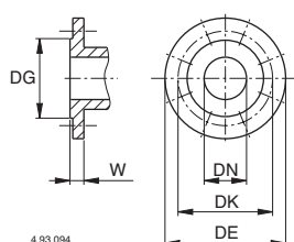
Flanges EN 1092-2
